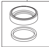
RP77552▲ Trim Ring and Gasket Aro de Accesorio y Empaque Anneau de finition et Joint
