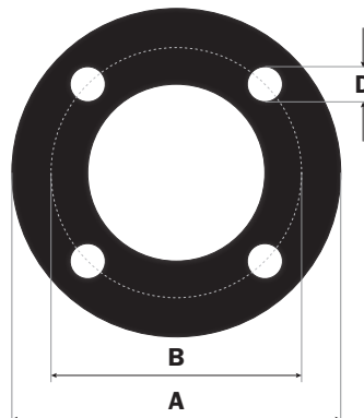
RF400 FLANGE
